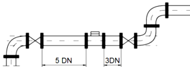
Рис. 3 Схема встановлення лічильника води
